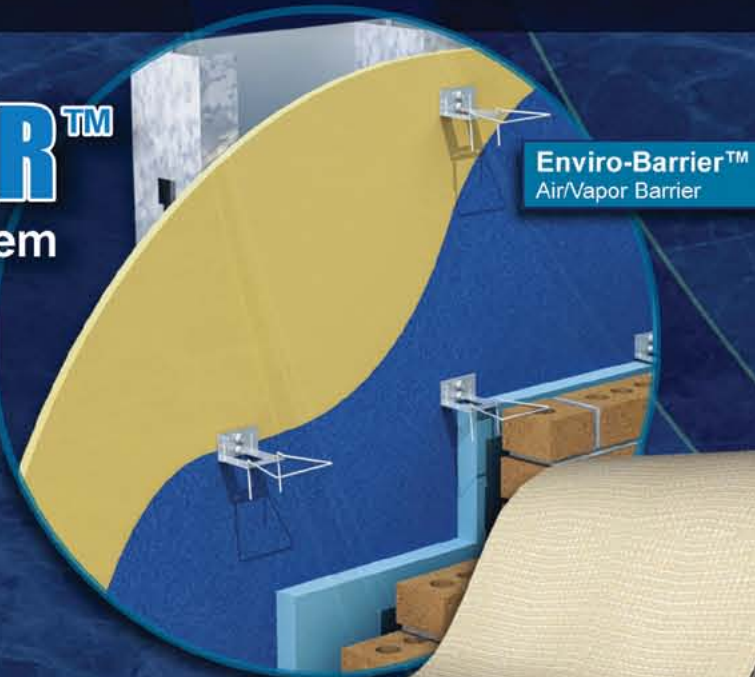
Stretch-X-Seal™ Window Pan Flashing
